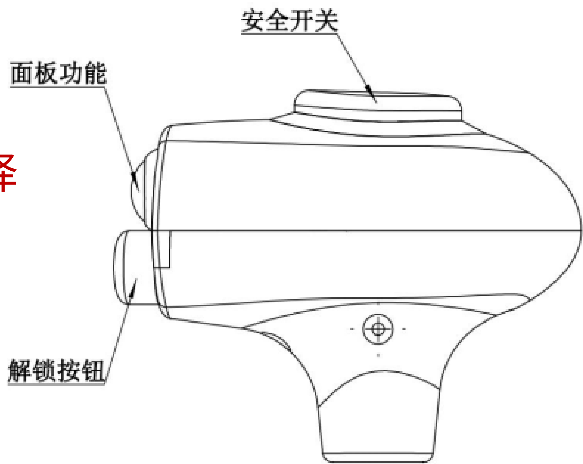
外形尺寸图
