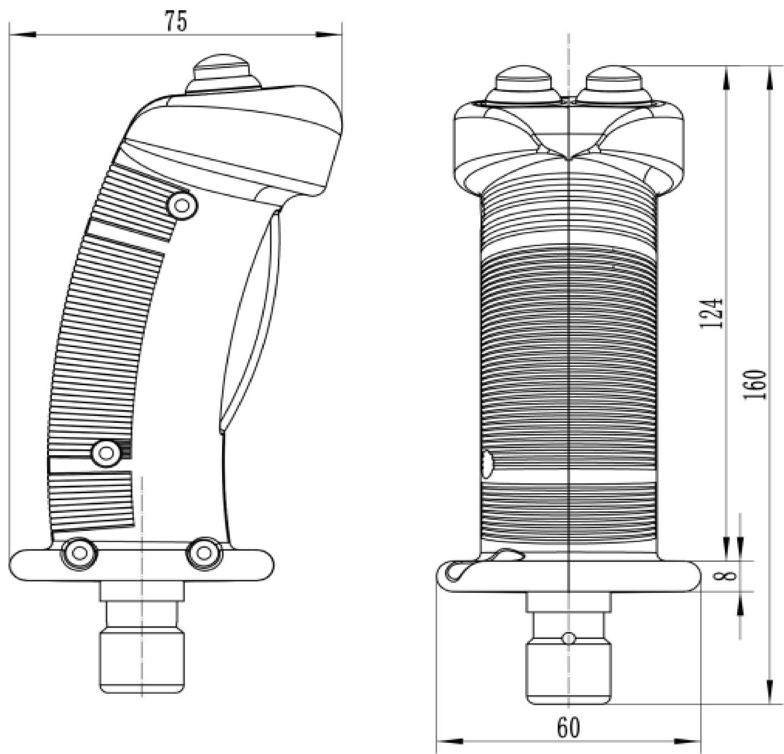
外形尺寸图
