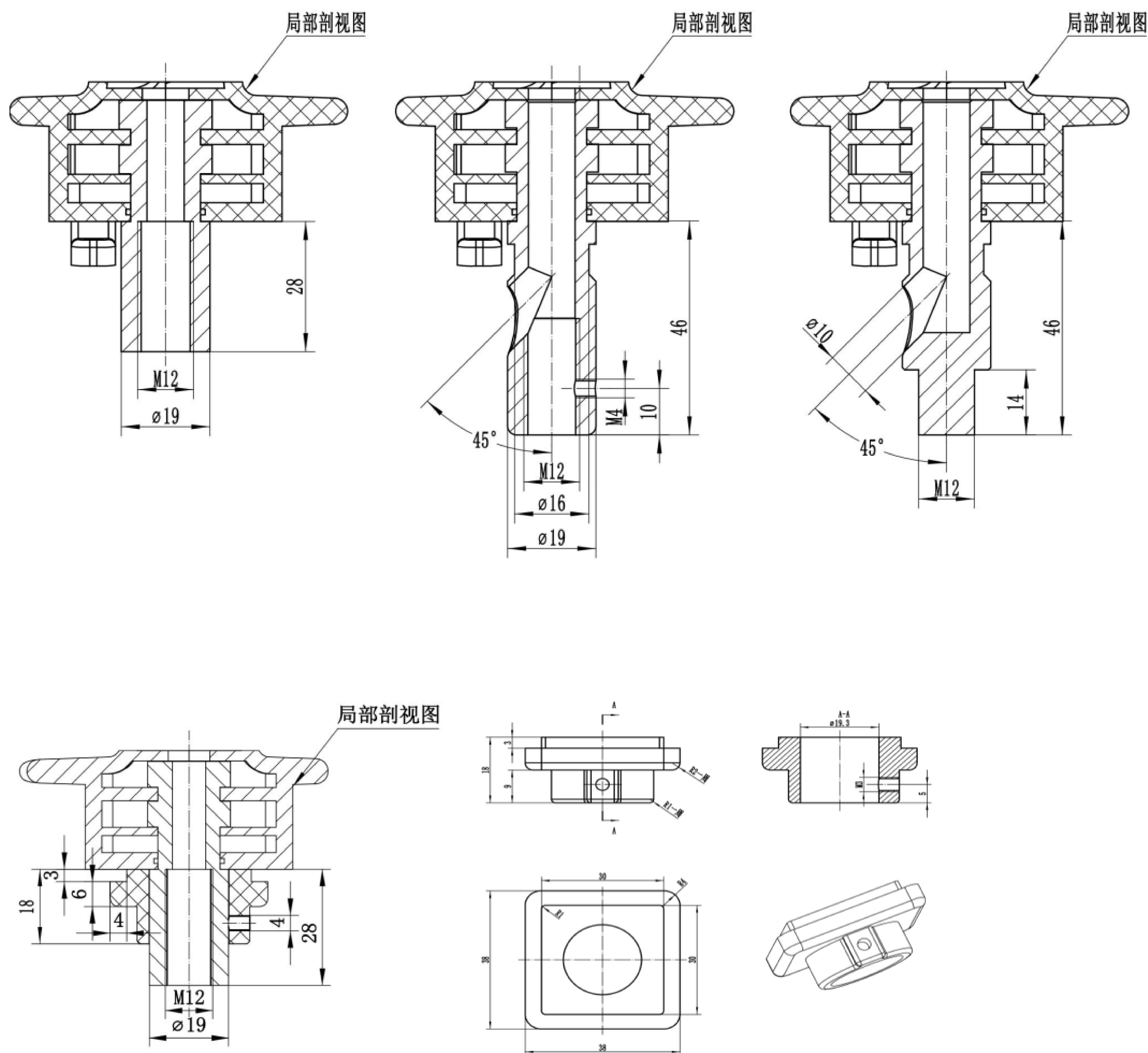
方形防尘套配件安装示意图
