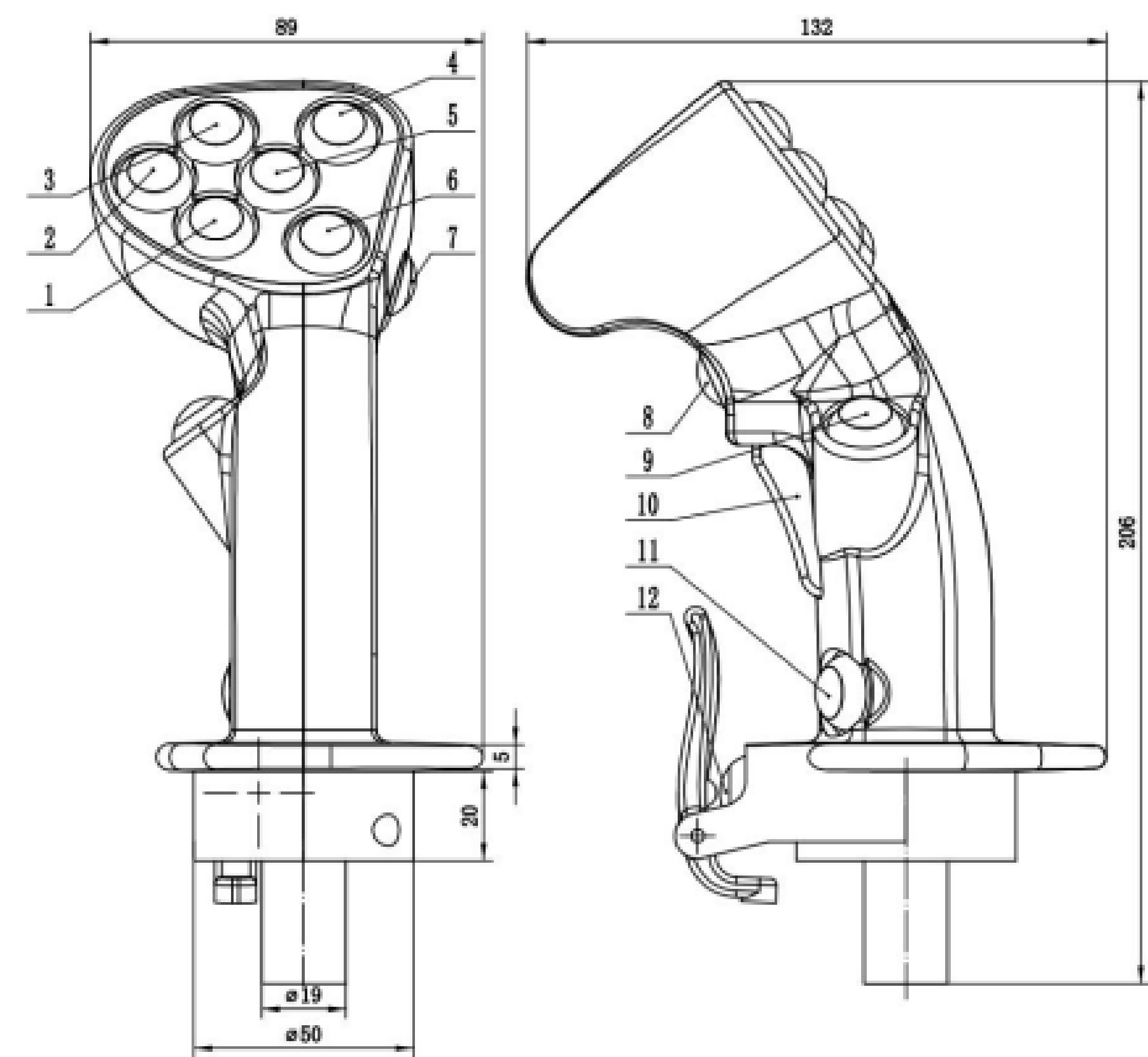
外形尺寸图
