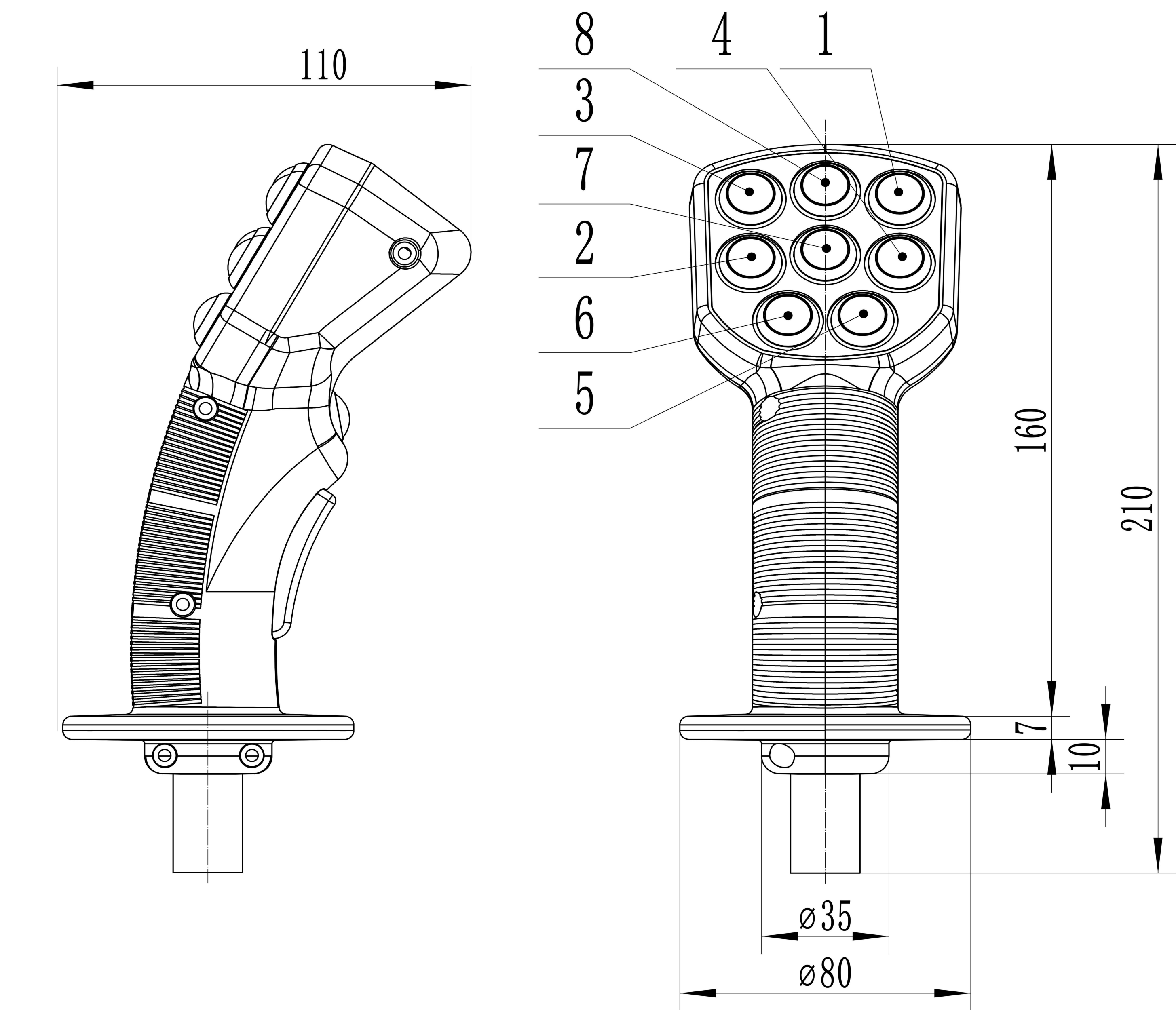
外形尺寸图
