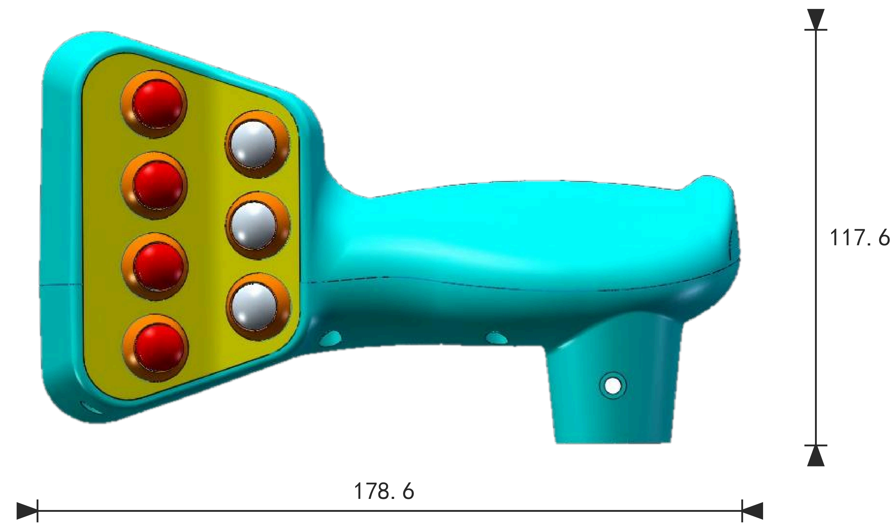
外形尺寸图（单位：mm）
